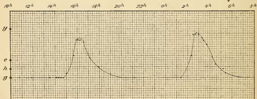
Lichtkurve von RW Draconis. (87. 1906.)
