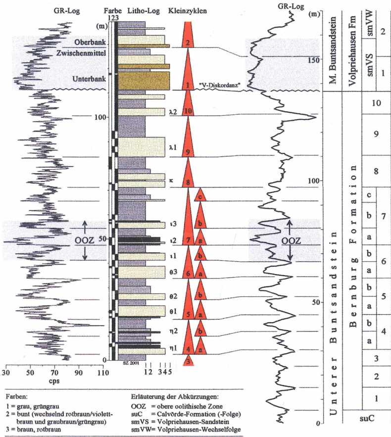
Abb.1: Vereinfachtes Profil der Aufschlüsse am Südhang des Marienburger Schloss- berges mit den Kleinzyklen 3-10 (orange Pfeile) der Bernburg-Formation (-Folge) sowie der Kleinzyklen 1-2 der Volpriehausen-Formation (-Folge). Vergleich des mit der Heger-Sonde erstellten Gamma-Ray-Logs (in cps, Impulse pro Sekunde) mit dem Gamma-Ray-Log der Bohrung Bockenem 1 (aus BOIGK 1959); Abbildung verändert aus SZURLIES (2001). Verwitterungsprofil: 1 = Tonsiltstein, 2 = Tonsiltstein-Feinsandstein Wechsellagerung, 3 = oolithischer Kalkstein, z.T. sandig, 4 = Feinsandstein, 5 = Mittel- und Grobsandstein.
