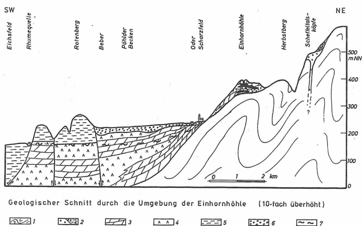
Abb. 8 Schematischer geologischer Schnitt durch die Umgebung der Einhornhöhle und Rekonstruktion der Landoberfläche vor Beginn des Quartärs. 1 = Grauwacken; 2 = permische Rhyolithe und Sedimente; 3 = Zechstein-Karbonate; 4 = Zechstein-Sulfate, 5 = Ton- und Schluffsteine des Zechsteins und Unteren Buntsandsteins; 6 = quartäre Schotter; 7 = Lage des Grundwasserspiegels im Zechstein-Aquifer. Nach VLADI (1984)
