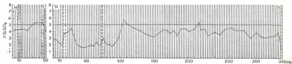
Abb. 5: Diagramm über Barytmächtigkeiten und \text{SrSO}_4 -Gehalte an der Aufschlußwand; Tagebau Königsgrube (aus: Stoppel & Gundlach 1972)
