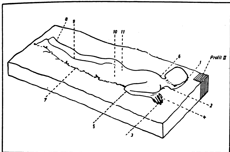
Abb. 4. Lage der Moorleiche von 1936 und Entnahmestellen von Untersuchungsproben
