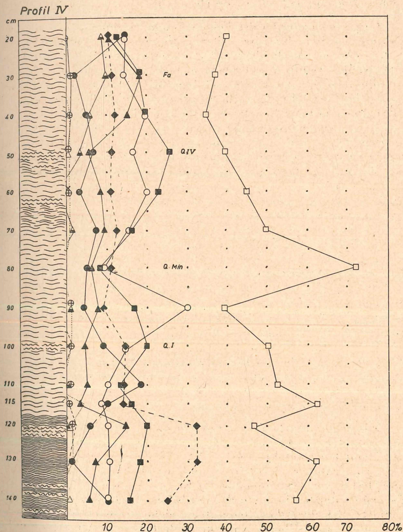
Abb. 6b. Pollendiagramm, 8 m westlich des Moorleichenfundes von 1931 entnommen
