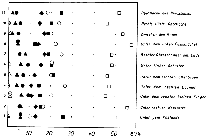
Abb. 5. Pollenspektren der Untersuchungsproben laut Abb. 4
