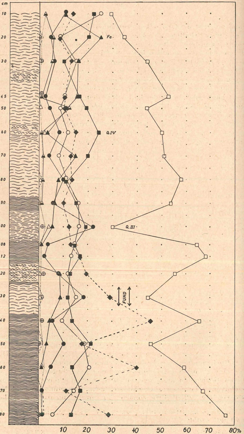
Abb. 6a. Pollendiagramm von der Fundstelle der Moorleiche von 1931
