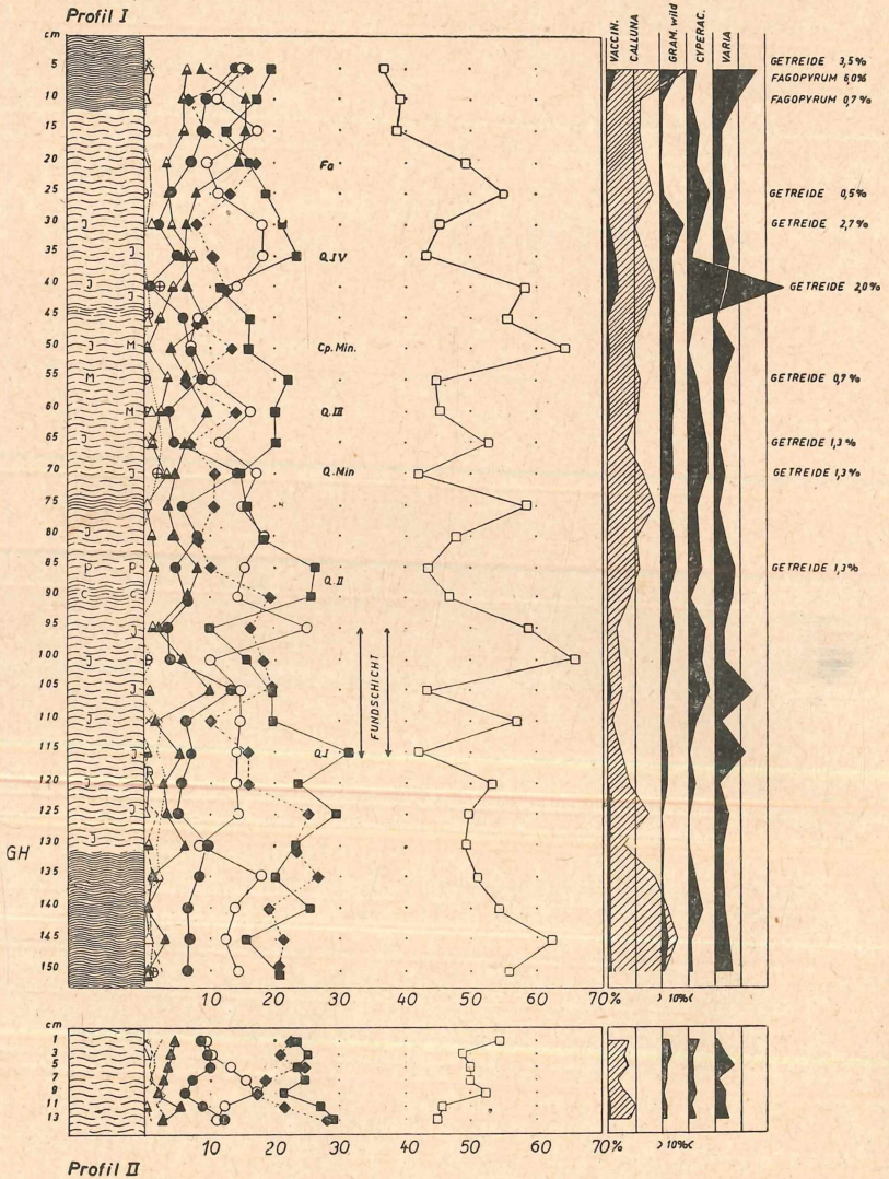
Abb. 3. Profil I: Pollendiagramm von der Fundstelle der Moorleiche von 1936. Profil II: Pollendiagramm eines Profils der Torfunterlage der Leiche (vergl. Abb. 4)
