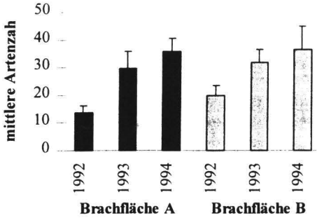
Abb. 2: Veränderung der mittl. Artenzahl auf den Brachflächen A und B (1992 Acker + 1994 Brache)
