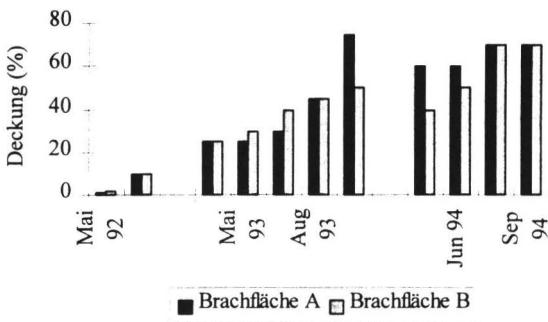
Abb. 1: Veränderungen der Vegetationsdeckung auf den Brachflächen A und B
