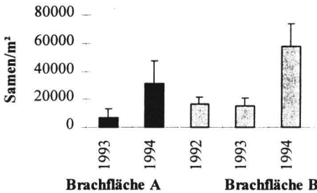
Abb. 3: Veränderung der mittleren Samendichte an den Intensivmeßpunkten auf den Brachflächen A und B (1992 Acker + 1994 Brache).
