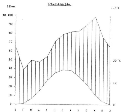
Abb. 2: Klimadiagramm (erstellt nach Daten der Meßstation Schwesing von 1961-1990, mit Genehmigung des Deutschen Wetterdienstes, Schleswig)
