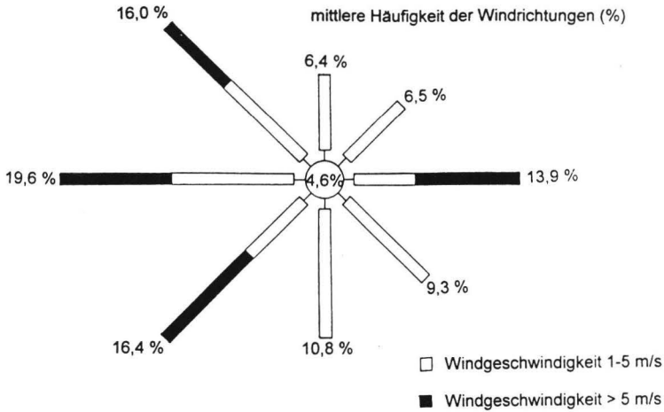
Abb. 3: Windrose (erstellt nach Daten der Meßstation Eggebek von 1973-1990). mit Genehmigung des Deutschen Wetterdienstes. Schleswig.
