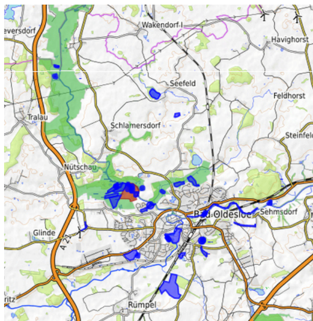
Abb. 10: Spießblättrige Melde Fundorte (in blau markiert) in Bad Oldesloe und Umgebung 2019–2022; rot: NSG Brenner Moor, grün: FFH-Gebiet Travetal (Karte aus Flora SH, 01.01.2023).
