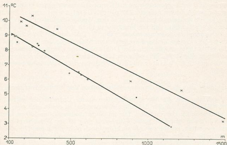
Abb. 1. Mittlere Jahrestemperatur in Abhängigkeit von der Höhenlage. Mittel der Jahre 1931 bis 1960. x Stationen des Südschwarzwaldes, o Stationen des Weserberglandes und des Harzes, (o) Station Witzenhäusen, nicht zur Berechnung der Regressionsgeraden mit herangezogen, ● Stationen der Rhön (Fulda, Wasserkuppe).
