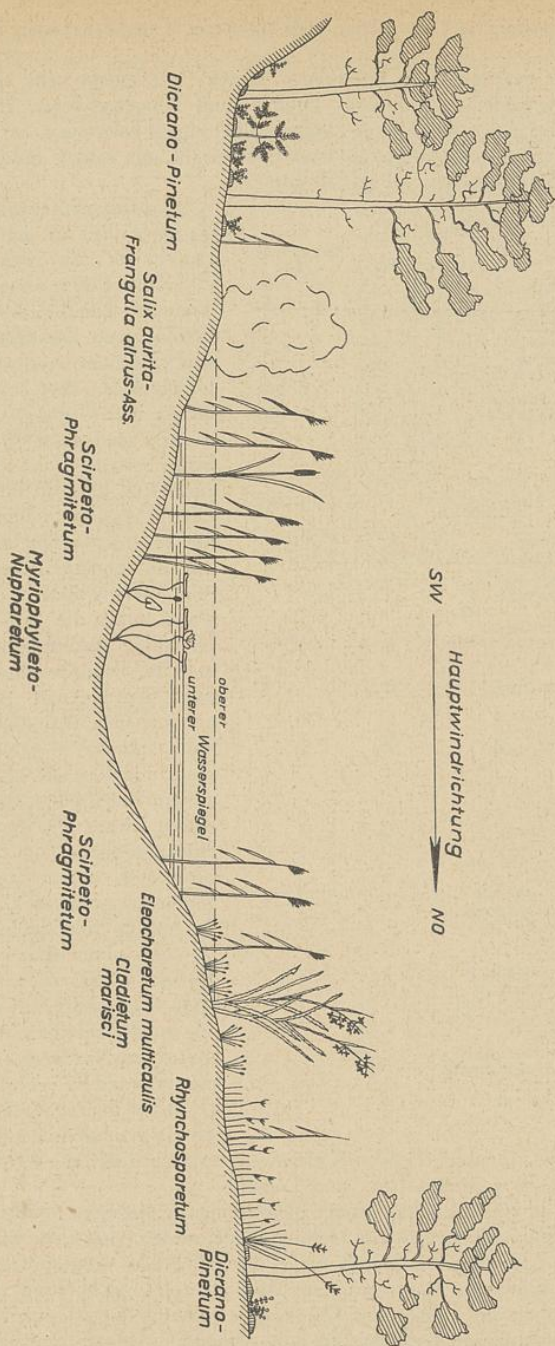
Vegetationsquerschnitt durch den Bräsen-See; links leeseitiges, rechts luvseitiges Ufer.
