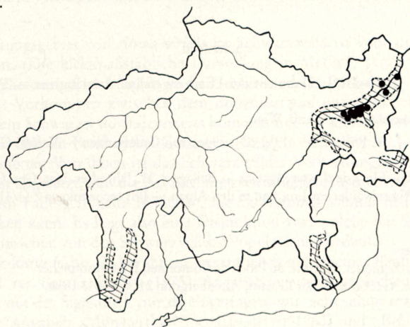
Abb. 2: Aufnahmestellen des Petasito-Cirsietum erisithalis im Unterengadin und das Areal von Cirsium erisithales in Graubünden
