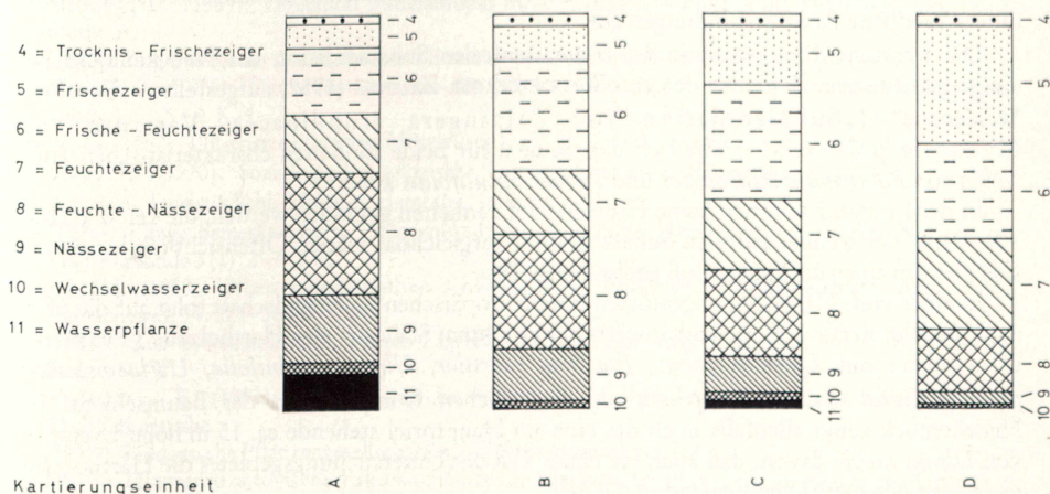
Abb. 2: Relativer Anteil der Zeiger verschiedener Feuchtegrade (n. ELLENBERG 1975) in den Kartierungseinheiten des Auenwaldes
