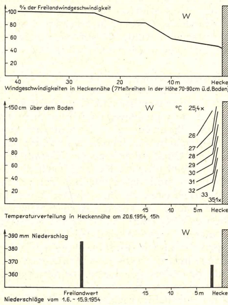
Abb. 4. Windgeschwindigkeit, Temperaturen und Niederschlag in Heckennähe (nach MÜLLER 1956).
