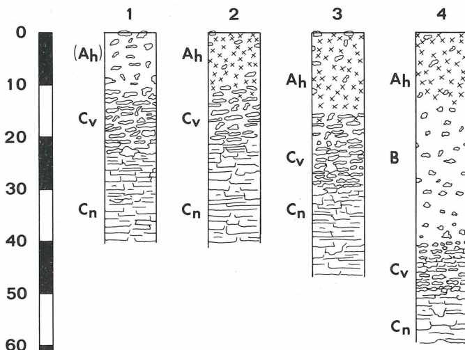
Abb. 3: Bodenprofiltypen der Kalk-Halbtrockenrasen am Kleinen Dörnberg.
