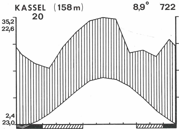
Abb. 2: Klimadiagramm der Wetterwarte Kassel für die 20jährige Meßperiode 1954–1973.
