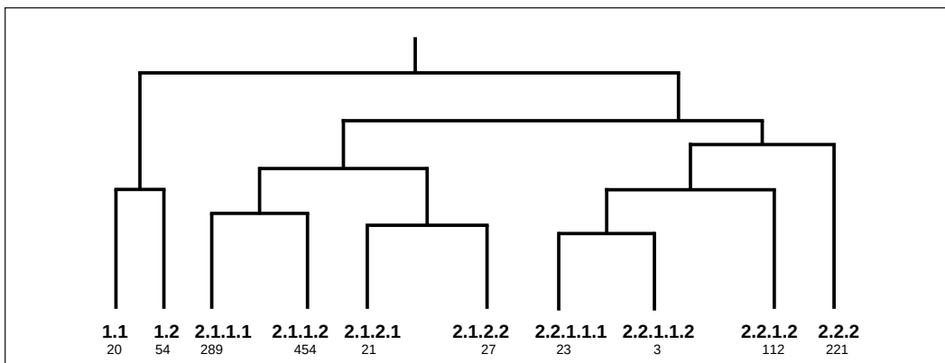
Abb. 5: Schematische Darstellung der 10-Cluster-Lösung des Complete-Linkage-Verfahrens. Die horizontalen Verbindungslinien geben keine Distanzen wieder, doch die vertikalen Verbindungslinien entsprechen schematisch proportional den zur Clusterzusammenführung (Verschmelzung) zu überwindenden Distanzen.
