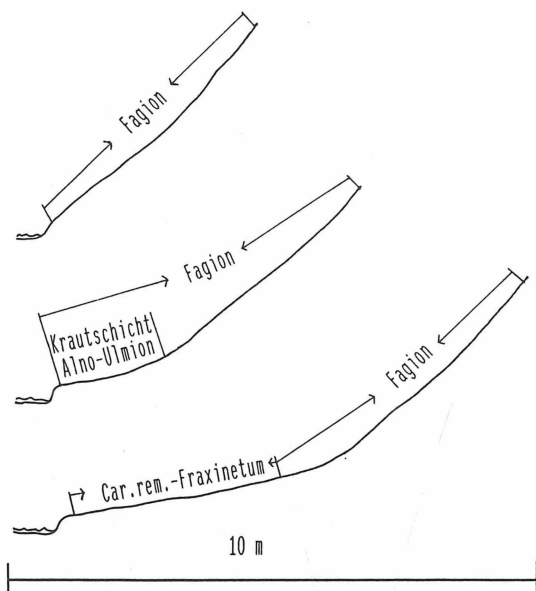
Abb. 7: Die typische Verknüpfung von den Pflanzengesellschaften Fagion und Carici remotae - Fraxinetum in den Kerbtälern des Ravensberger Hügellandes in Abhängigkeit von der Hangneigung, dargestellt an halbseitigen Geländeprofilen.
