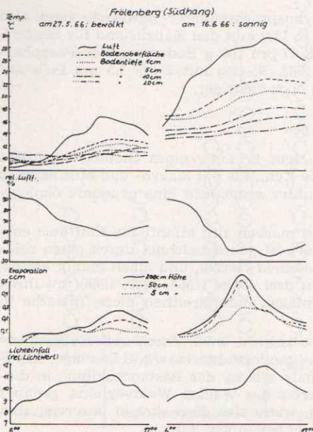
Abb. 5: Mikroklimatisches Diagramm zweier Meßtage vom S-Hang des Frölenberges
