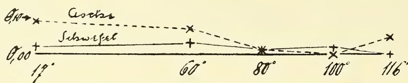
Fig. 11. Veränderung des Schwefel- und Aschegehalts mit der Temperaturzunahme.
