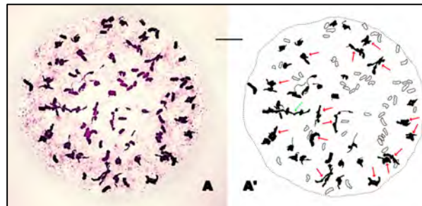
Fig. 9. Comportamiento meiótico en células madre de esporas (microfotografía y diagrama) de A. x sollerense (especimen n° 8): A- metafase I, n= c. 1 IV, 15 III, 23 II, 49 I, A'- diagrama explicativo: bivalentes, en negro; univalentes, perfilados; flechas rojas trivalentes; flecha verde tetravalente. La localidad de origen puede verse en el apéndice 1. Barra de escala 10 \mu\text{m} .
