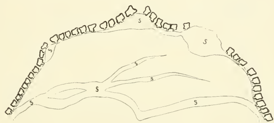
Fig. 6. — Péridermes superposés.
