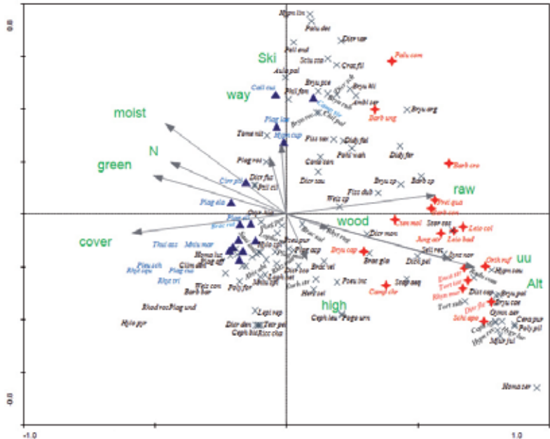
Abb. 4: Verteilung der Moosarten in einer Korrespondenzanalyse von 221 Aufnahmeplots. Blaue Dreiecke: Nutzungszeiger, rote Sterne: Natürlichkeitszeiger. Umweltparameter wurde als Zusatzinformation sekundär eingefügt. Abkürzungen: Alt = Seehöhe, cover = Vegetationsdeckung, green = Grünland, high = Vegetationshöhe, moist = Bodenfeuchte, N = mittlere Stickstoffzahl, raw = Rohhumus, Ski = Schipiste, uu = ungenutzte Flächen, way = Weg, wood = Forst. Moosnamen sind eindeutig abgekürzt; x = Ubiquisten und seltene Arten. Eigenwert der ersten und zweiten Achse 0.764 und 0.551, Summe der kanonischen Eigenwerte 2.668.
