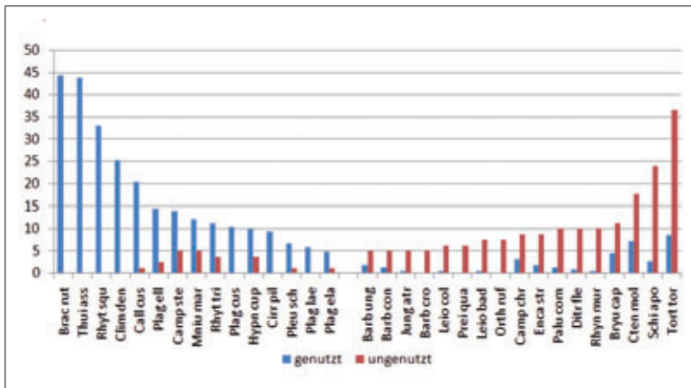
Abb. 3: Verteilung der Moos-Arten ab 5 % Frequenzanteil (Y-Achse) am jeweiligen Nutzungstyp nach Nutzung bzw. Nichtnutzung innerhalb der 1-m 2 -Plots. Links (getrennt durch ein leeres Feld) die Arten, die mehr als doppelt so oft auf genutzten Flächen vorkommen als auf ungenutzten, rechts mehr als doppelt so oft in ungenutzten Flächen. Artnamen eindeutig abgekürzt (siehe auch Text).
