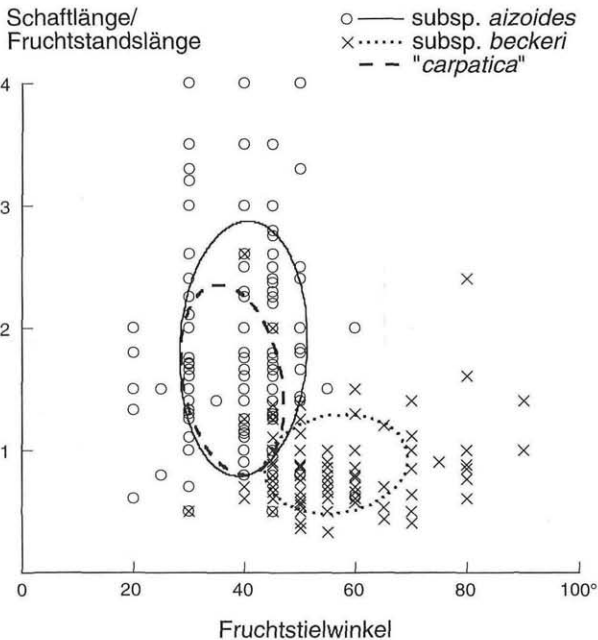
Abb. 3. Draba aizoides s. l., Korrelation der Verhältniszahlen Schaftlänge : Fruchtstandslänge zu den Fruchtsielwinkeln. Die Ellipsen umfassen jeweils 66% der Einzelwerte, die jeweils auf ein Individuum bezogen sind; die Einzelwerte von „ carpatica “ sind aufgrund der zahlreichen Überlappungen mit subsp. aizoides nicht gesondert dargestellt.
