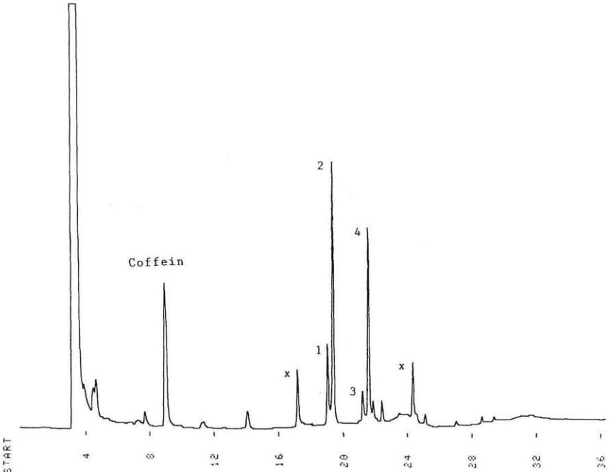
Abb. 2. Gaschromatogramm des Extraktes von Onosma alborosea (x: nichtalkaloidische Verunreinigung).
