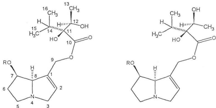
Abb. 1. Formeln der vier in Onosma gefundenen Pyrrolizidinalkaloide.
