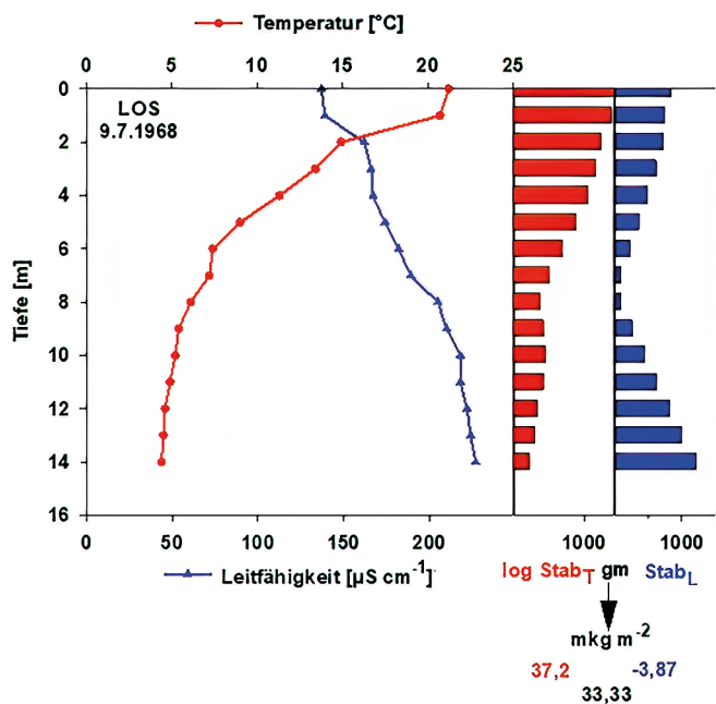
Abb. 7: Tiefenprofile für Temperatur und Leitfähigkeit am 9. Juli 1968 im Lunzer Obersee (LOS) und die daraus berechnete Tiefenverteilung der thermischen ( Stab_T ) und der Konzentrations-Stabilität ( Stab_L ), sowie die sich ergebende Gesamtstabilität der Wassersäule. Aus Daten in den Protokollheften im Nachlass Berger. – Fig. 7: Depth profiles for temperature and conductivity on 9 July 1968 in Lunzer Obersee (LOS) and the calculated depth distribution of the thermal ( Stab_T ) and the concentration stability ( Stab_L ), as well as the resulting overall stability of the water column. From data in the booklets of Berger's legacy.
