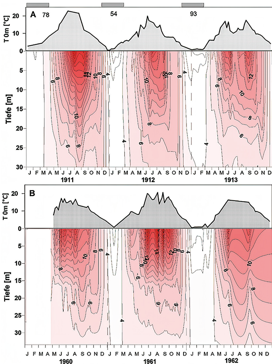
Abb. 16: Lunzer Untersee. A. Jahresgänge der Oberflächentemperatur ( T_{0m} ) und Tiefen-Isolinien der Wassertemperatur beide in ^{\circ}C für die Jahre 1911 bis 1913 nach Daten in Ruttner (1930). Die Dauer der Vereisung sind als graue Flächen angegeben und darunter als Dauer in Tagen. B. Jahresgänge der Oberflächentemperatur ( T_{0m} ) und Tiefen-Isolinien der Wassertemperatur für die Jahre 1960 bis 1962 nach Daten aus dem Nachlass Berger, Protokollheft Heigl. Vereisungsdaten waren darin nicht verzeichnet. – Fig. 16: Lunzer Untersee. A. Annual cycles of surface water temperature ( T_{0m} ) and depth isopleths of water temperature both in ^{\circ}C for the years 1911 to 1913 according to data in Ruttner (1930). The duration of the ice cover is indicated in gray and below in days. B. Annual cycles of surface water temperature ( T_{0m} ) and depth isopleths of water temperature for the years 1960 to 1962 according to data from the Berger legacy, protocol book Heigl. Ice data were not recorded.
