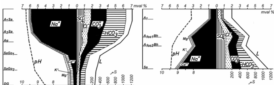
Abb. 1: Konzentration an löslichen Ionen, Leitfähigkeit (in Mikrosiemens – \mu\text{S} ) und pH in Solontschak-Solonetz (Sk-Sz; links, Salz im Oberboden) und Solonetz (Sz; rechts, Salz im Unterboden). Sk-Sz: wie beim typischen Sk bildet Sa den Oberboden, jedoch leicht überdeckt von ebenfalls sehr salzreichem Sediment. Sz: über Schotter liegt der salzführende Horizont (Sa), darüber der humose A-Horizont (A ...) als Folge spätglazialer und holozäner Bodenbildungen (aus GHOBADIAN 1966, verändert; dort nähere bodenkdl. Details). – Fig. 1: Concentrations of soluble ions, conductivity (microsiemens – \mu\text{S} ) and pH in solonchak-solonetz (Sk-Sz; left, salt in the topsoil) and solonetz (Sz; right, salt in the subsoil). Sk-Sz: as for typical Sk, Sa forms the topsoil layer, but is shallowly covered with sediments as saline as the Sa itself. Sz: the saline horizon (Sa) lies over gravel being covered with a humus-rich A-horizon (A ...) as a result of soil formations during late Glacial and/or Holocene periods (from GHOBADIAN 1966, modified).
