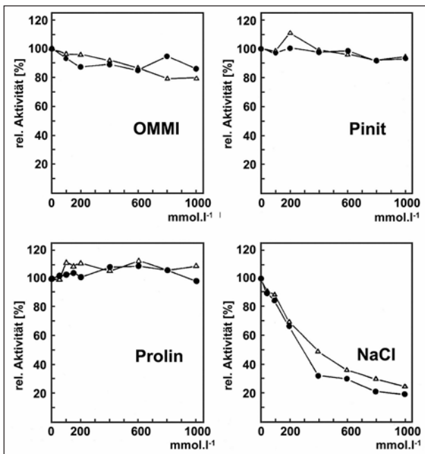
Abb. 6: Wirkung unterschiedlicher Konzentrationen von zugesetztem OMMI (= 1D-1-O-methyl-muco-Inositol), Pinit, Prolin und NaCl auf die Malatdehydrogenase in Blättern von Rhizophora mangle . Dreiecke: Pflanzen in 10 % Meerwasser, Kreise: Pflanzen in 100 % Meerwasser (aus SOMMER et al. 1990, verändert). – Fig. 6: Effect of OMMI (1D-1-O-methyl-muco-inositol), pinitol, proline and NaCl at various concentrations on malate dehydrogenase activity of Rhizophora mangle leaves. Triangles: leaves of plants grown in 10 % sea water, dots: leaves of plants grown in 100 % sea water (from SOMMER et al. 1990, modified).
