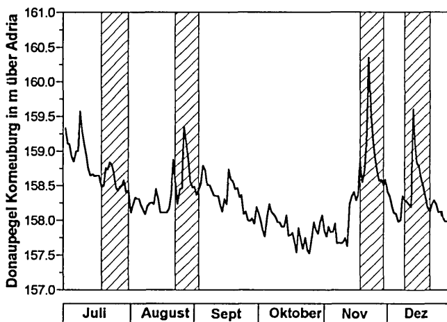
Abb. 2: Donaupegel Korneuburg von Juli bis Dezember 1994. Die Probentermine sowie die Expositionsdauer der künstlichen Substrate sind schraffiert hinterlegt. – Water level at Korneuburg from July to December 1994. Sampling dates and exposition times of artificial substrata are hatched.
