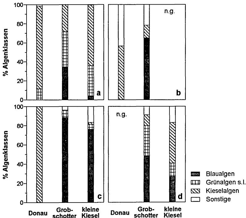
Abb. 3: Verteilung der Algenklassen auf Donauschotter (alle Punkte miteinbezogen) und im Phytoplankton auf der Basis der HPLC-Analyse: (a) 18.7., (b) 22.8., (c) 17.11., (d) 8.12. Abk.: n.g. = nicht gemessen. — Algal class-composition on gravel (all sampling points are considered) and in phytoplankton of the Danube River analyzed by means of HPLC: (a) July 18 th , (b) August 22 nd , (c) November 17 th , (d) December 8 th . Abbreviation: n.g. = not measured).
