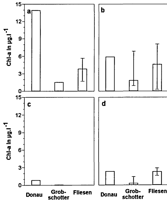
Abb. 5: Mediane/Extremwerte von Chl-a auf künstlichen Substraten und im Pelagial, alle Punkte miteinbezogen. Chl-a in \mu\text{g}\cdot\text{l}^{-1} (Donau) bzw. \mu\text{g}\cdot\text{cm}^{-2} (Benthos): (a) 31.7., (b) 2.9., (c) 30.11., (d) 20.12. Abk.: n.g. = nicht gemessen. — Medians/extremes of Chl-a on artificial substrates and in the pelagial; all sampling locations are considered: (a) July 31 st , (b) September 2 nd , (c) November 30 th , (d) December 20 th ). Abbreviation: n.g. = not measured).
