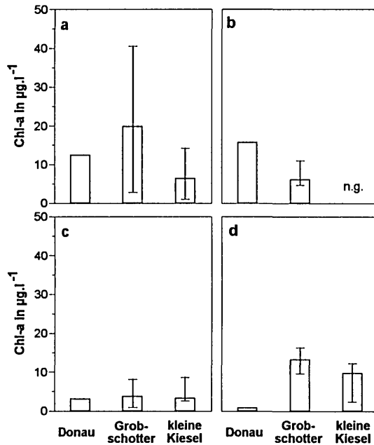
Abb. 4: Mediane/Extremwerte von Chl-a auf natürlichem Substrat und im Pelagial, alle Punkte miteinbezogen. Chl-a in \mu\text{g}\cdot\text{l}^{-1} (Donau) bzw. \mu\text{g}\cdot\text{cm}^{-2} (Benthos): (a) 18.7., (b) 22.8., (c) 17.11., (d) 8.12. Abk.: n.g = nicht gemessen. – Medians/extremes of Chl-a on natural substrate and in the pelagial; all sampling locations are considered: (a) July 18 th , (b) August 22 nd , (c) November 17 th , (d) December 8 th ). Abbreviation: n.g. = not measured).
