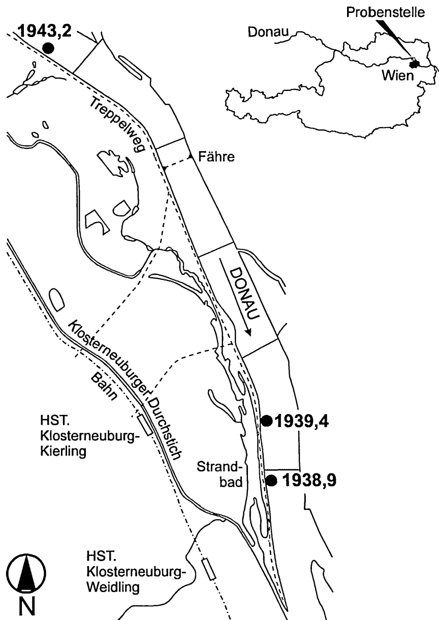
Abb. 1: Untersuchungsgebiet bei Klosterneuburg, Lage der Probenpunkte. — Investigation area and sampling points near Klosterneuburg.
