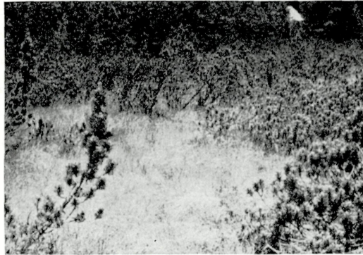
Abb. 3. Hochmoor „Große Kohlstatt“. Eriophoro-Sphagnetum recurvi inselartig im Sphagno-Mugetum entwickelt.
