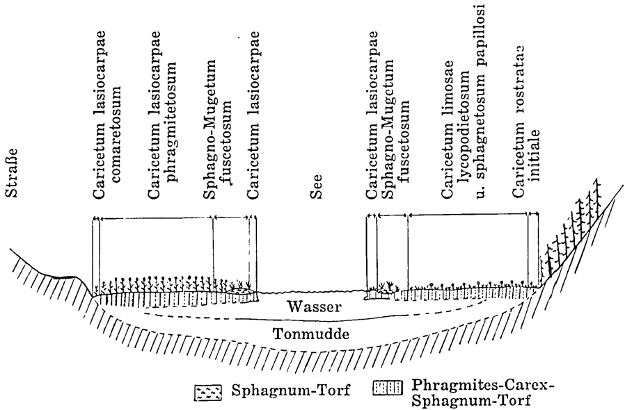
Abb. 1. Querschnitt durch den Ostteil des Moores am Seethaler See (schematisch).
