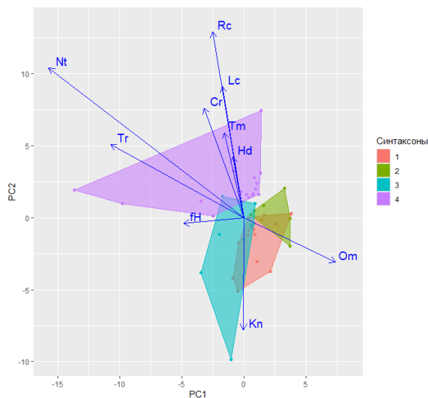
Рис. 5. PCA-ординация синтаксонов.
