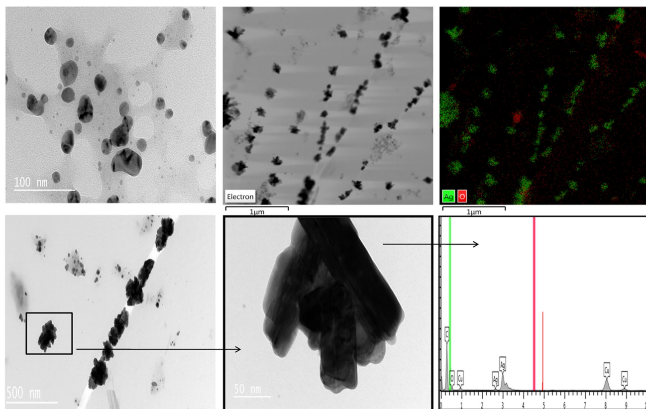
Fig. 1 TEM images of HA-AgNPs
