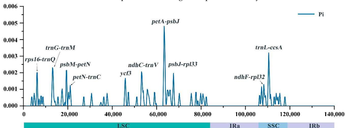
Figure 5. Nucleotide diversity (Pi) based on sliding window analysis in the aligned complete chloroplast genomes of S. spontaneum , S. officinarum , S. robustum , S. sinense , S. barberi , and S. hybrids .
