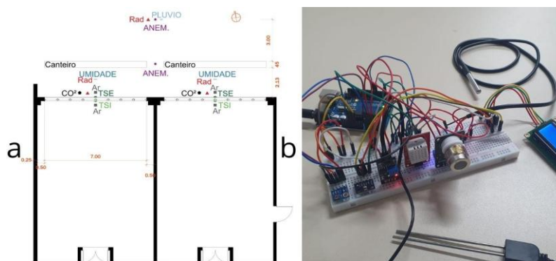
Figura 5: Posicionamento e calibração dos sensores.
