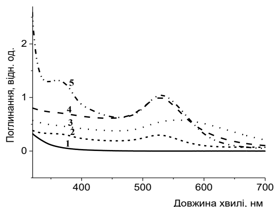
Рис. 4. Спектри поглинання: 1 – прекурсор HAuCl_4 , 2 – зразок №2 AuНЧ-танін + K_2CO_3 , 3 – зразок №4 AuНЧ-алое (в.е.), 4 – зразок №3 AuНЧ-алое (с.е.), 5 – зразок №1 AuНЧ-танін
