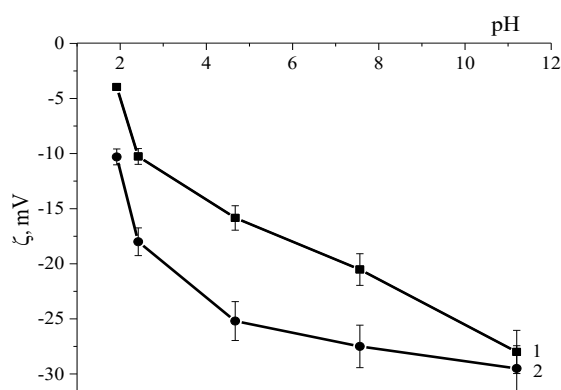
Рис. 1. Залежність електрокінетичного потенціалу (ζ) наночастинок срібла, синтезованих за допомогою спиртового екстракту евкаліпту (1) та розчину таніну (2), від величини pH водного розчину
