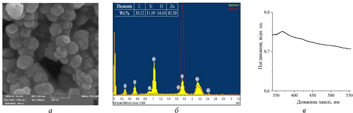
Рис. 6. СЕМ-зображення (а), EDX спектр, елементний аналіз (б) і спектр поглинання (в) наночастинок оксиду цинку синтезованих із застосуванням спиртового екстракту квітів нагідок
