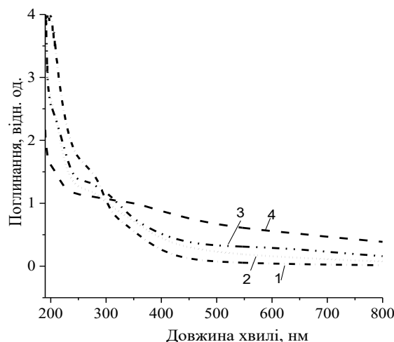
Рис. 5. Спектри поглинання: 1 – прекурсор \text{FeCl}_3 , 2 – зразок №4 \text{Fe}_x\text{O}_y\text{НЧ} -гібіскус (в.е.), 3 – зразок №1 \text{Fe}_x\text{O}_y\text{НЧ} -кропива (в.е.), 4 – зразок №2 \text{Fe}_x\text{O}_y\text{НЧ} -іван-чай, 5 – зразок №3 \text{Fe}_x\text{O}_y\text{НЧ} -подорожник (в.е.)
