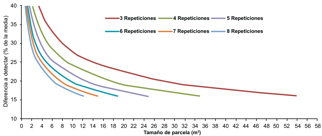
Figura 5. Relación entre tamaño de parcela, número de repeticiones y diferencia verdadera a detectar en un experimento de frijol.
