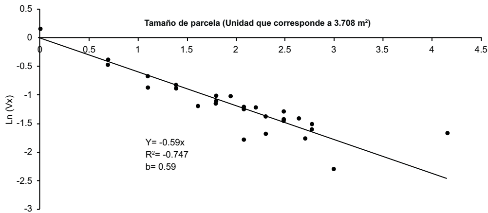
Figura 3. Regresión lineal del logaritmo de la varianza del rendimiento (Vx) en función del logaritmo del tamaño de parcela (x).
