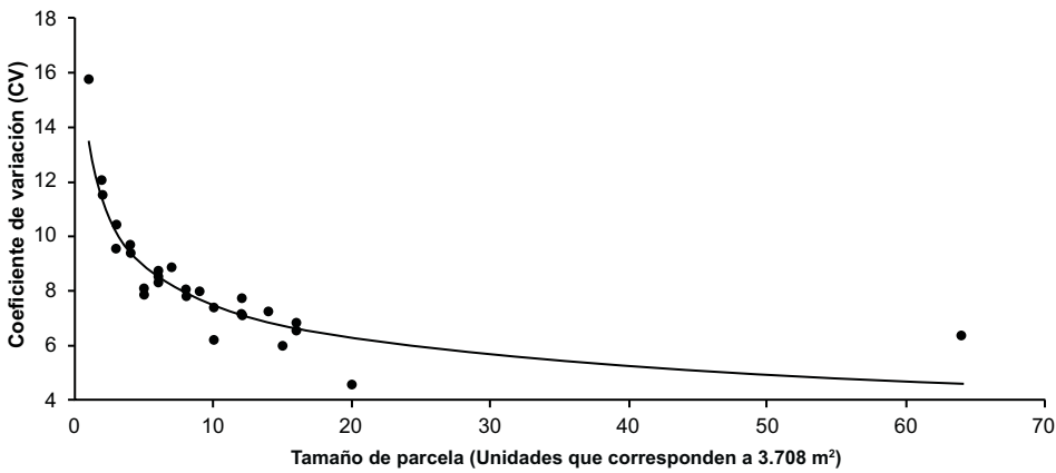
Figura 4. Relación entre el coeficiente de variación (CV) del rendimiento y la unidad de parcela.
