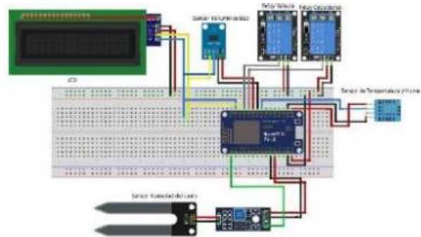
Fig. 7. Diseño del circuito para controlar el cultivo invernadero.
