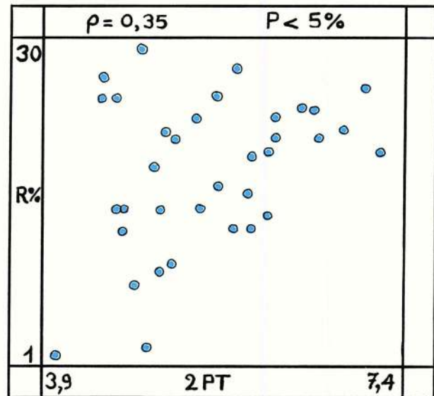
FIG. 10. — Corrélation entre l'épaisseur et le retrait de la double paroi, pour 35 parois d'Ekoune.
