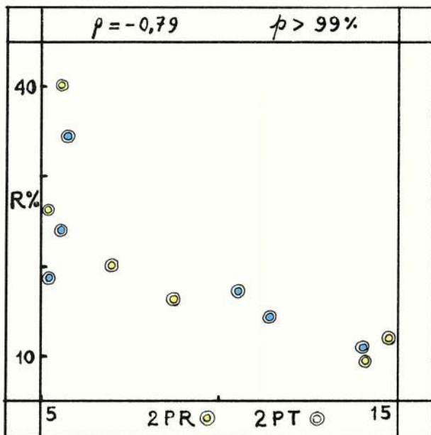
FIG. 9. — Corrélation entre l'épaisseur et le retrait de la double paroi, pour les moyennes de chaque éprouvette.
