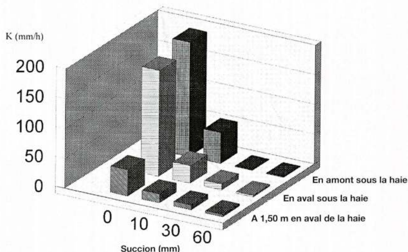
Figure 2. Conductivité de l'horizon A d'un andosol au voisinage d'une haie de Calliandra calothyrsus et sous différentes succions contrôlées.
