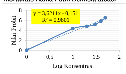
Diagram 2. Grafik Analisis Probit Mortalitas Hama Putih Bemisia tabaci
