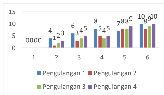
Diagram 1. Grafik Mortalitas Hama Bemisia tabaci setiap Perlakuan
